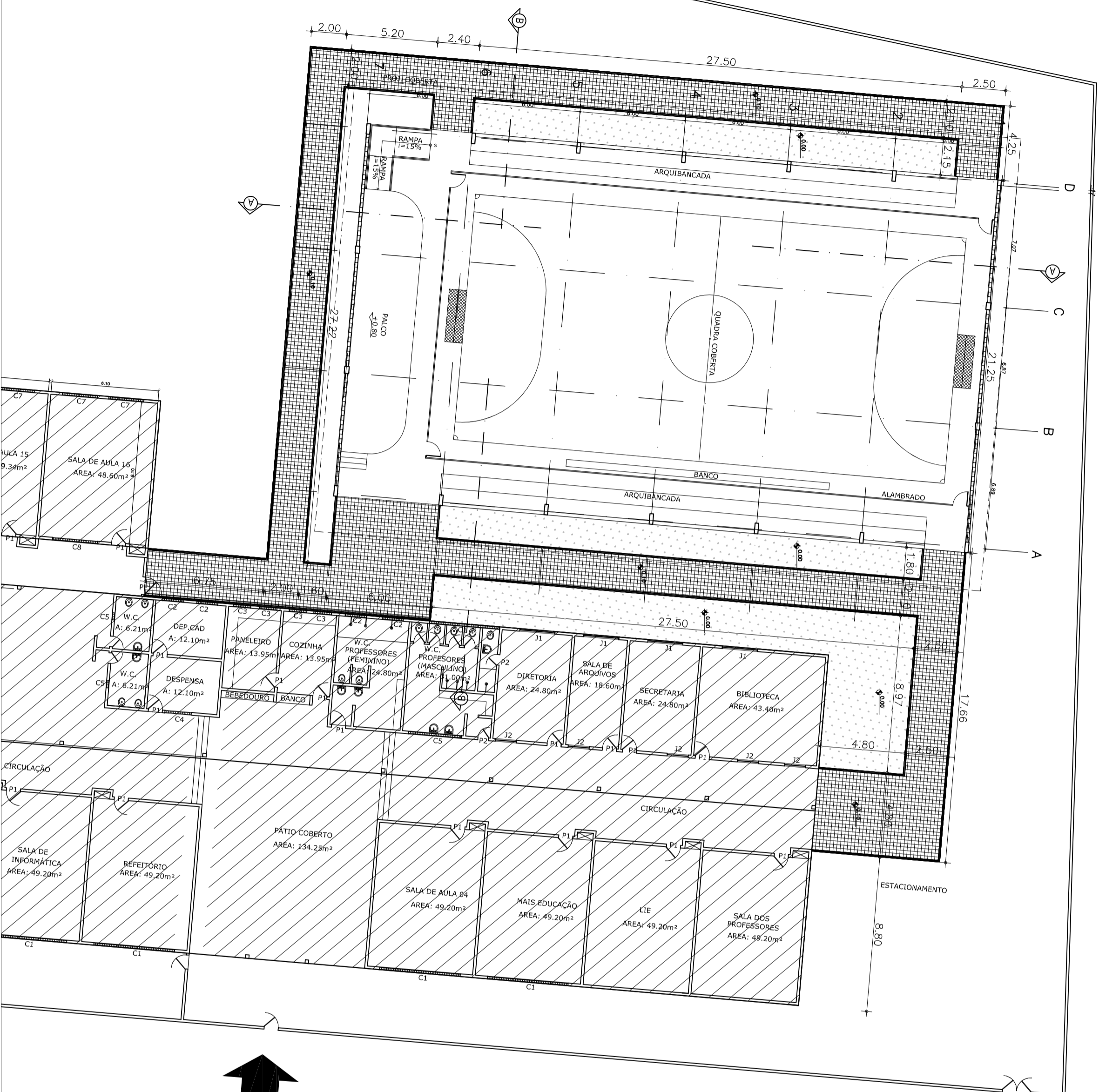
1 PLANTA DE LOCAÇÃO DOS PILARES ESC.: 1:200
